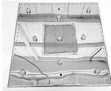
Imagem 1 (Base Inox)
